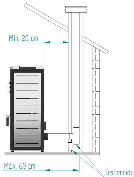
Figura 18 - Vista lateral de la instalación con chimenea, con ejemplo del punto de inspección
