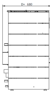
Figura 2 - Dimensiones de la estufa de pellets Douro 12 kW
