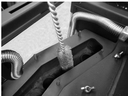
Figura 41 - Limpieza de los canales de paso de aire y turbuladores
