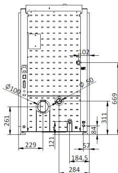
Figura 4 - Dimensiones de la estufa de pellets Douro 23 kW
