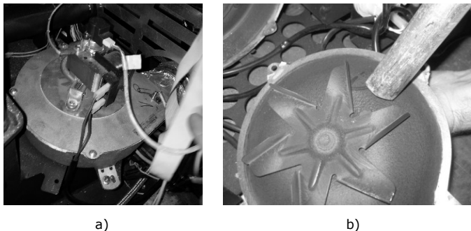
Figura 39 - Aspirar el área del paso de aire
