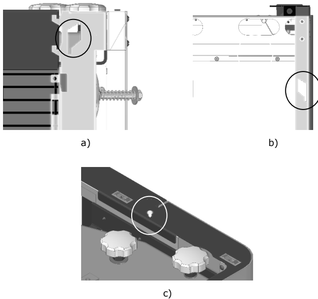
Figura 12 - Envolvente Douro 12 kW
