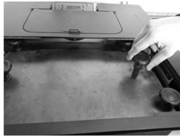
Figura 30 - Limpieza de los turbuladores
