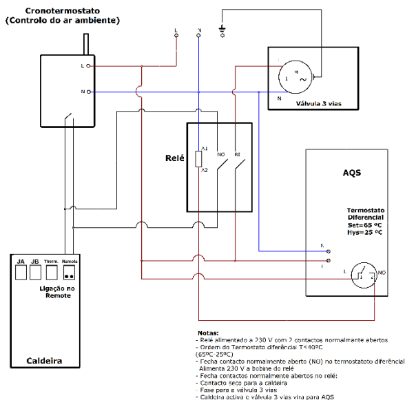
Figura 49 - Conexión eléctrica de un cronotermostato (Control del aire ambiente) de un termostato diferencial conectado al tanque de agua caliente y la válvula de tres vías para una caja de relés
