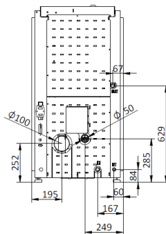
Figura 3 - Dimensiones de la estufa de pellets Douro 17 kW
