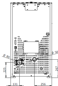
Figura 2 - Dimensiones de la estufa de pellets Douro 12 kW
