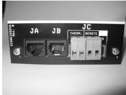
Figura 26 - Mando externo (cronotermostato) e interfaz de conexão – ambos no incluídos
