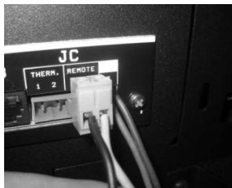
Figura 27 - Conexión del mando remoto inalámbrico
