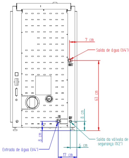
Figura 6 – Ligações hidráulicas da salamandra a pellets (Douro 17 kW)
