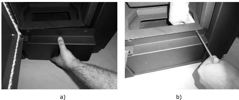
Figura 14 - Montagem da capa frontal inferior
