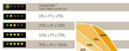
Figura 57 - Níveis de performance da bomba
