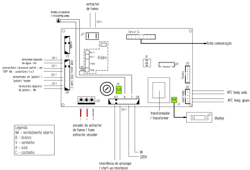
Figura 53 - Esquema eléctrico Douro 12 kW
