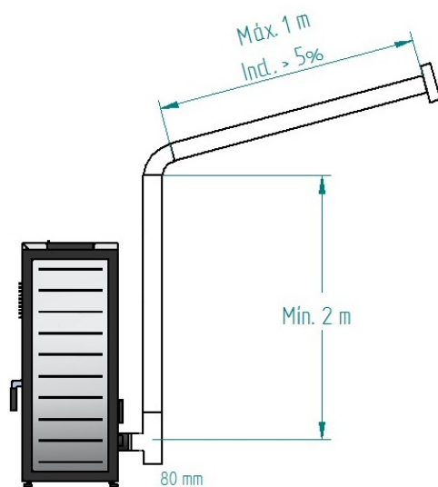
Figura 17 – Exemplos de instalações tipo
