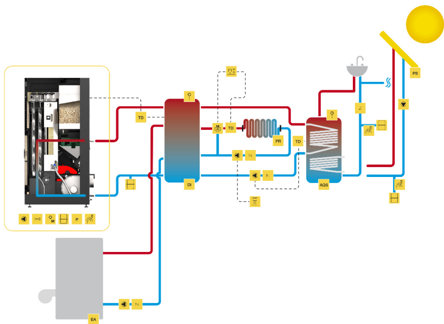
Figura 51 - Ligação a chão radiante, conjugado com outra caldeira de apoio e águas sanitárias combinado com painel solar
