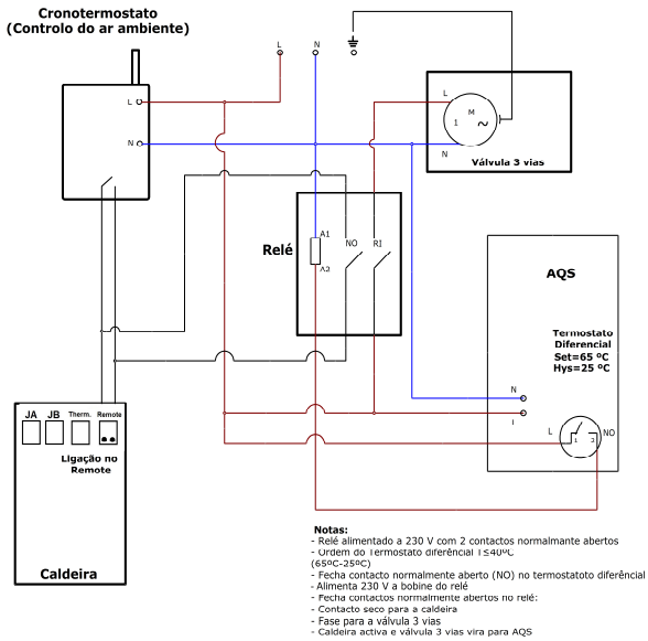
Figura 49 - Ligação eléctrica de um cronotermostato (controlo do ar ambiente) de um termostato diferencial ligado ao depósito de AQS e da válvula de três vias a uma caixa de relés
