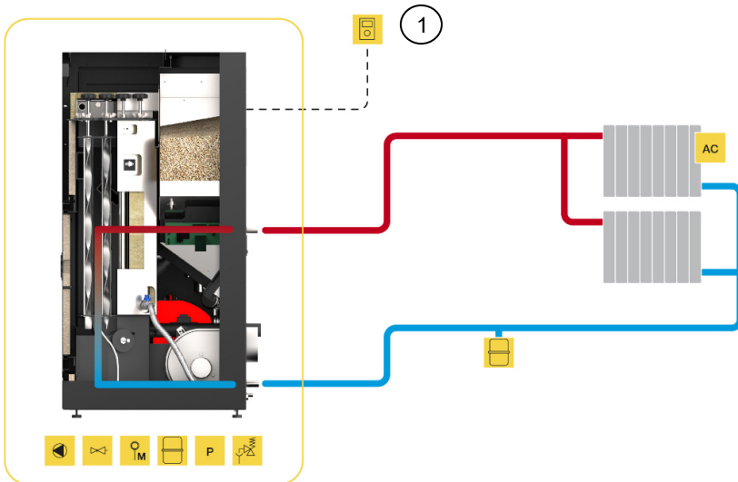
Figura 47 - Ligação simples apenas a radiadores de aquecimento central
