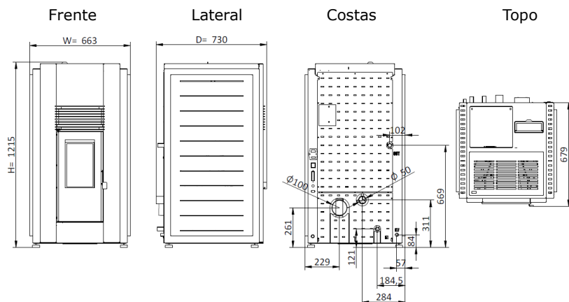
Figura 4 - Dimensões da salamandra a pellets (Douro 23 kW)
