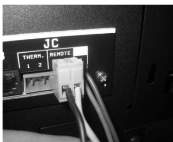
Figura 27 - Ligação do comando remoto sem fios
