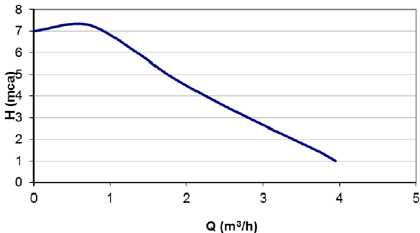
Figura 55 - Gráfico de desempenho da bomba
