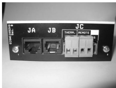
Figura 26 - Comando externo (cronotermostato) e interface de ligação – ambos não incluídos
