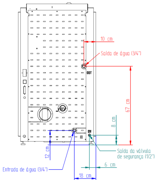
Figura 7 – Ligações hidráulicas da salamandra a pellets (Douro 23 kW)
