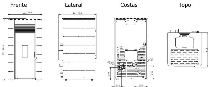
Figura 2 - Dimensões da salamandra a pellets (Douro 12 kW)
