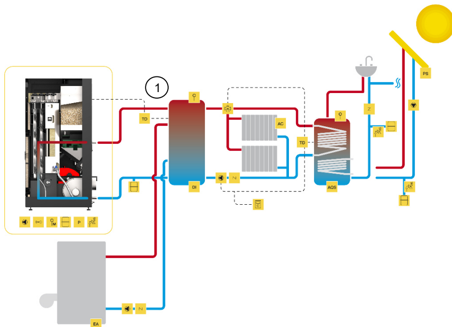
Figura 50 - Ligação a radiadores de aquecimento central, conjugado com outra caldeira de apoio e águas sanitárias combinado com painel solar
