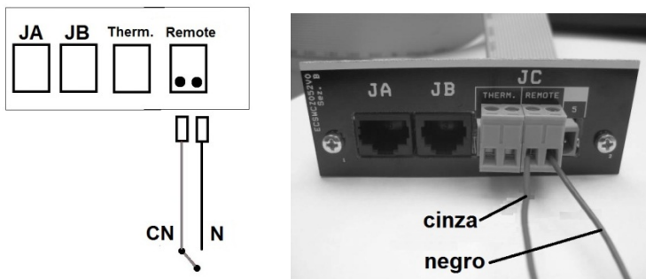
Figura 28 - Ligações do comando externo com fios
