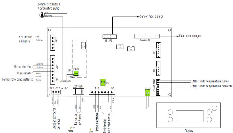
Figura 54 - Esquema eléctrico Douro 17 kW e 23 kW
