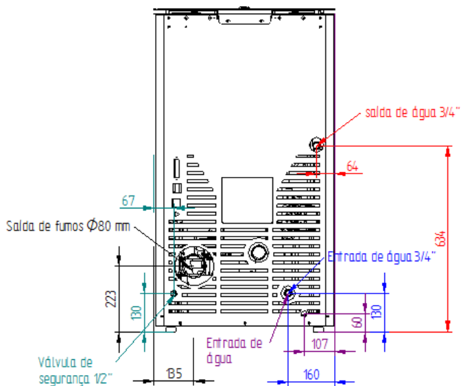
Figura 5 – Ligações hidráulicas da salamandra a pellets (Douro 12 kW)
