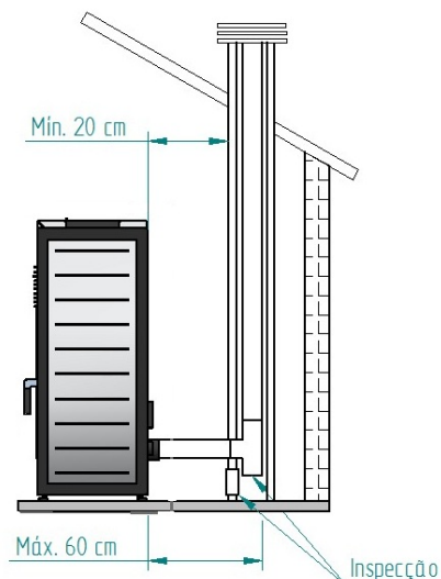
Figura 18 – Vista lateral da instalação com chaminé, com exemplo do ponto de inspeção
