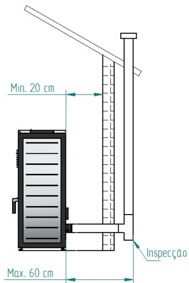
Figura 16 – Vista lateral da instalação sem chaminé, com exemplo do ponto de inspeção
