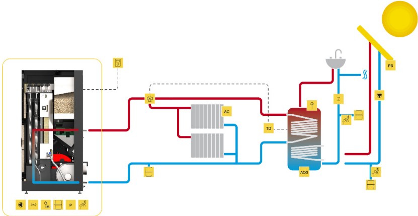
Figura 48 - Ligação a radiadores de aquecimento central e águas sanitárias combinado com painel solar
