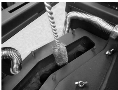
Figura 41 - Limpeza dos canais de passagem de ar e turbuladores
