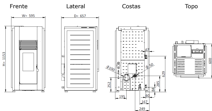
Figura 3 – Dimensões da salamandra a pellets (Douro 17 kW)
