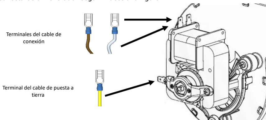
Figura 116 – Conexión de cableado al ventilador
