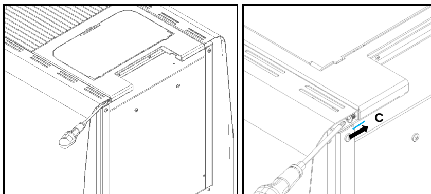
Figura 103 – Fijación de las envolventes
