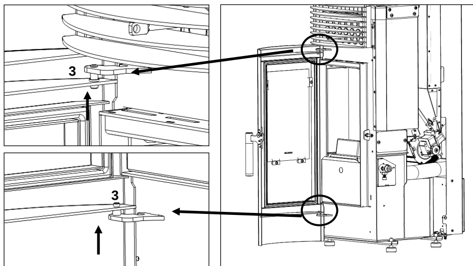
Figura 75 - Desmontaje de la puerta
