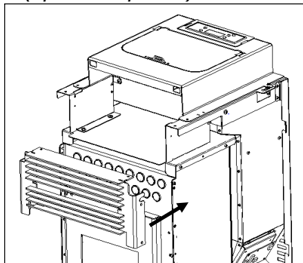
Figura 56 - Apretar la rejilla frontal
