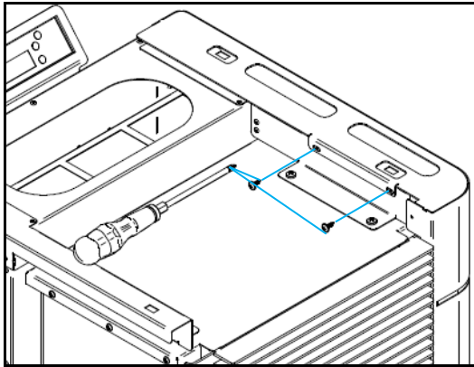
Figura 22 - Fijación de las laterales de las envolturas na parte superior
