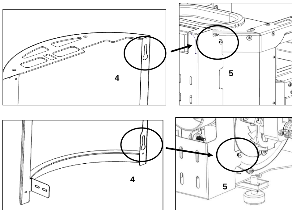
Figura 77 - Montaje de la tapa lateral
