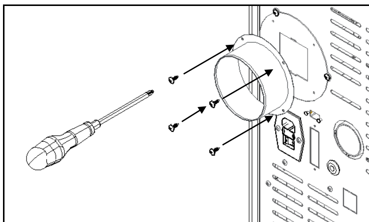
Figura 130 - Colocación de la boca de salida de aire en la estufa
