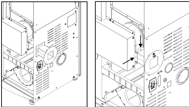
Figura 128 - Colocación de la guía de aire en la estufa
