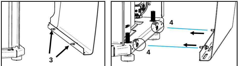
Figura 39 - Fijación de las envolventes Pine e Leaf
