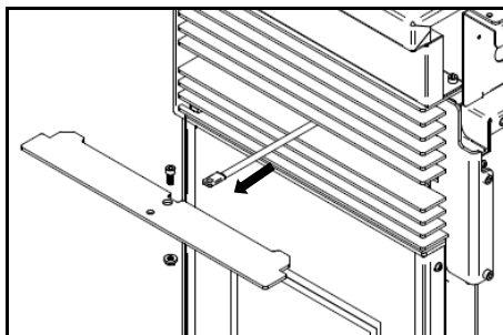
Figura 57 - Apretar la pala de registro
