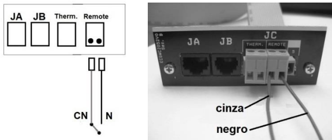
Figura 147 – Conexiones del mando externo con cables
