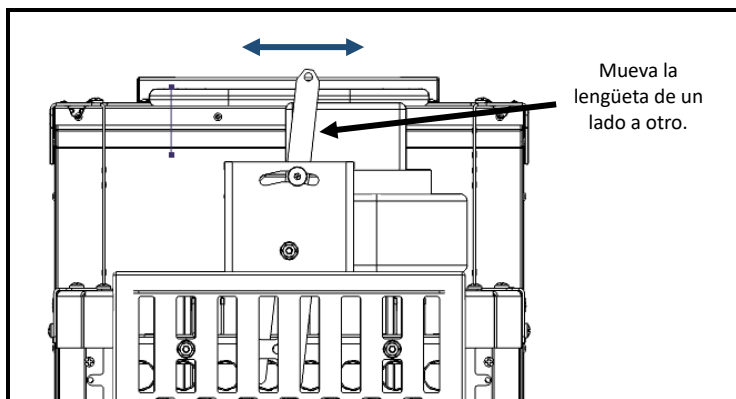
Figura 117 – Comprueba el bloqueo
