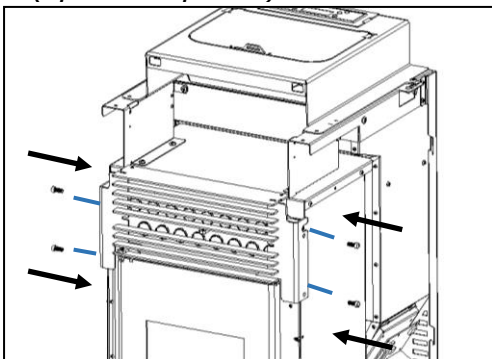
Figura 56 - Apretar la rejilla frontal
