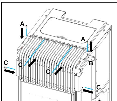
Figura 86 – Apriete de la rejilla frontal
