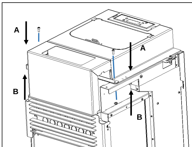
Figura 60 – Apretar la frontal del acabamiento del equipo Alpes K400
