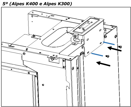
Figura 52 - Fijación de la pantalla en la posición correcta en la estructura del equipo
