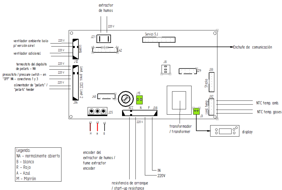
Figura 150 – Esquema eléctrico estufa K100, K200, K500 y K600
