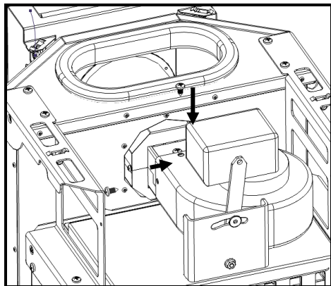
Figura 113 – Colocación de la guía de aire en la estufa
