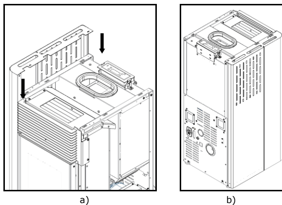
Figura 95 – Colocación de las envolventes laterales
