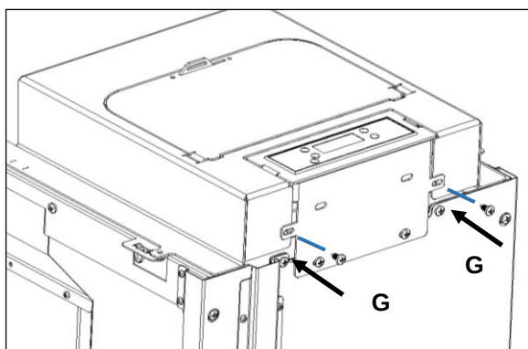
Figura 55 - Colocación de la tapa superior en la estructura del equipo
