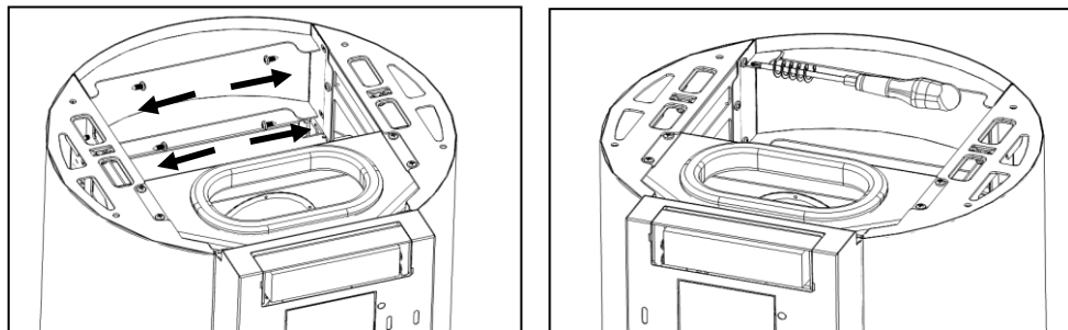
Figura 79 - Fijación de la tapa al frontal de acabado
