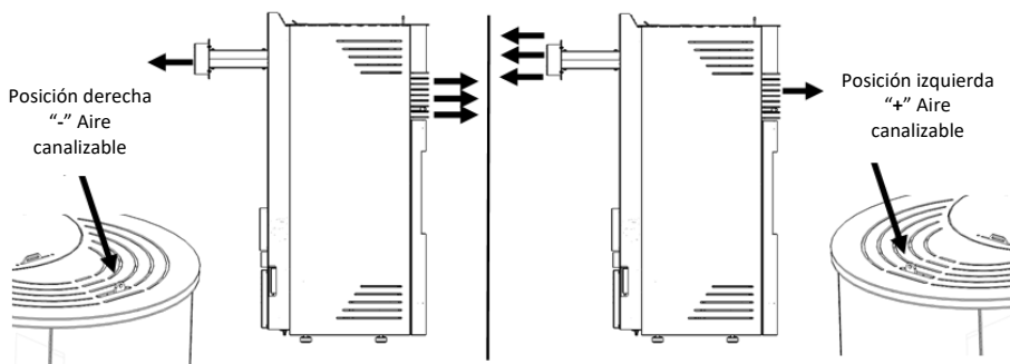
Figura 121 – Regulación del registro de aire canalizable “+” o “-”
