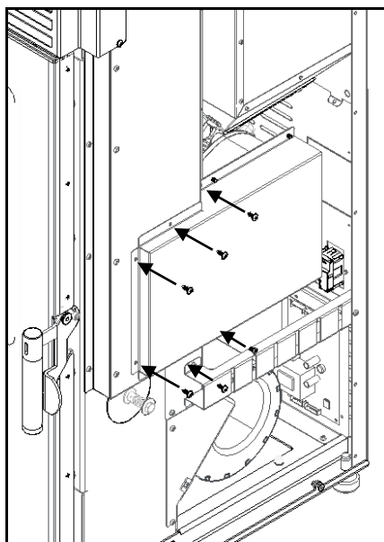
Figura 126 - Fijación del ventilador al equipo
