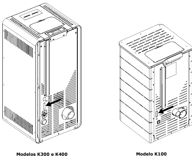
Figura 144 – Lugar donde se instala la placa interfaz
