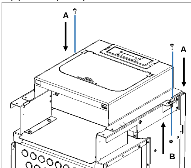
Figura 54 - Fijación de la tapa superior de la estructura del equipo
