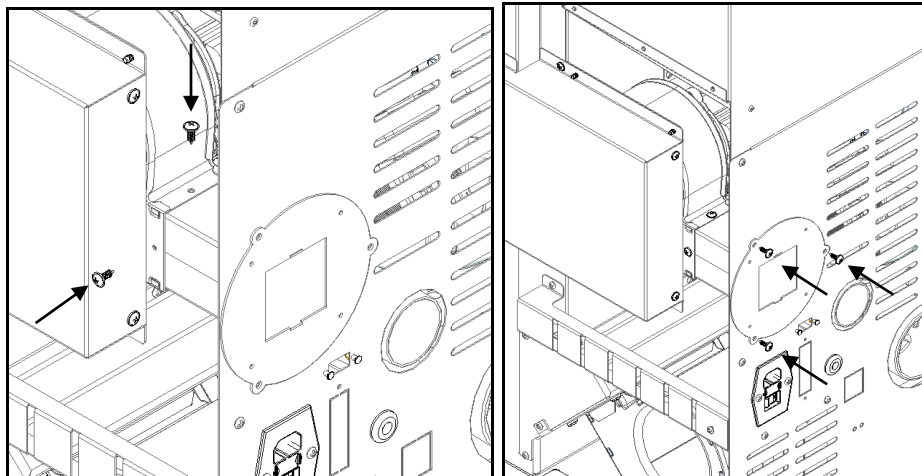
Figura 129 - Colocación de la guía de aire en la estufa
