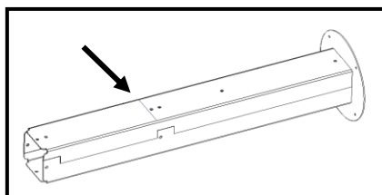
Figura 119 – Zona de corte de la parte "guía" del aire canalizado
