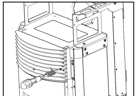
Figura 106 – Retirada de la rejilla
