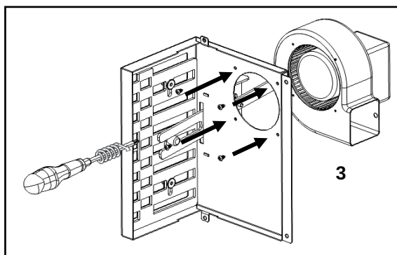
Figura 109 – Fijación del soporte con el ventilador
