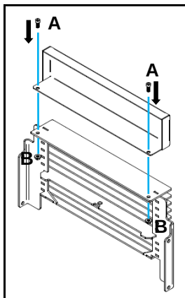
Figura 36 - La unión parrilla delantera con el tiro arriba
