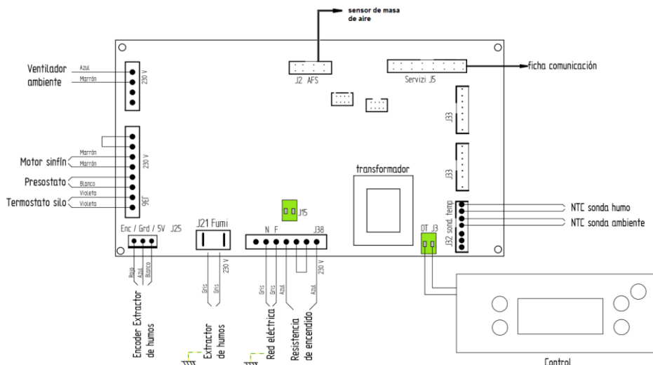
Figura 151 – Esquema eléctrico estufa K300 y K400
