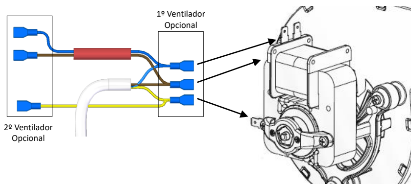
Figura 132 - Conexión de cableado al ventilador
