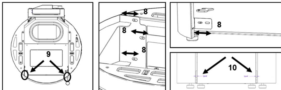
Figura 81 - Ajuste las tapas en el equipo
