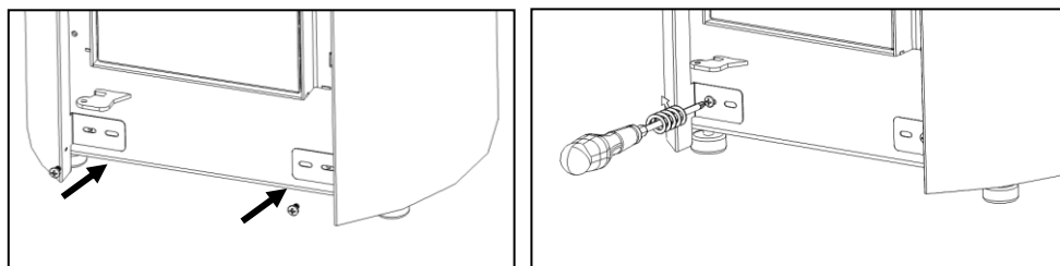
Figura 80 - Fijación de la tapa en la parte frontal del equipo
