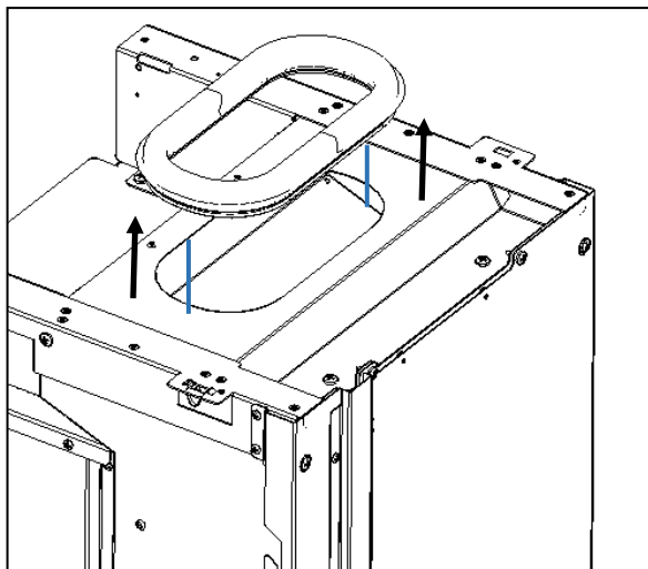
Figura 50 - La eliminación de la junta de goma en la máquina
