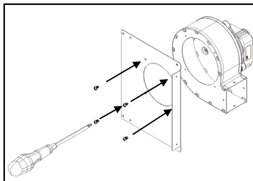
Figura 124 - Fijación del soporte con el ventilador
