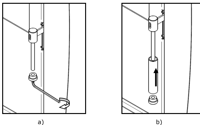
Figura 45 - Montaje de la manija
