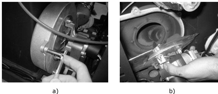
Figura 143 – a) Retirar los tornillos; b) Retirar el extractor
