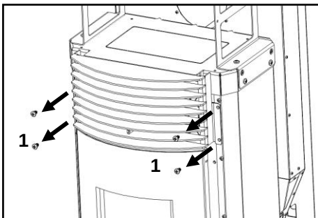
Figura 106 – Retirada de la rejilla
