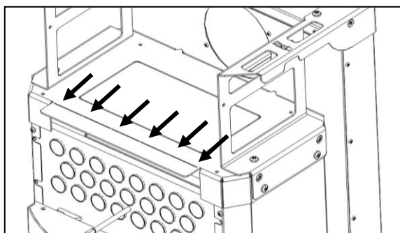
Figura 108 – Quitar la visera frontal
