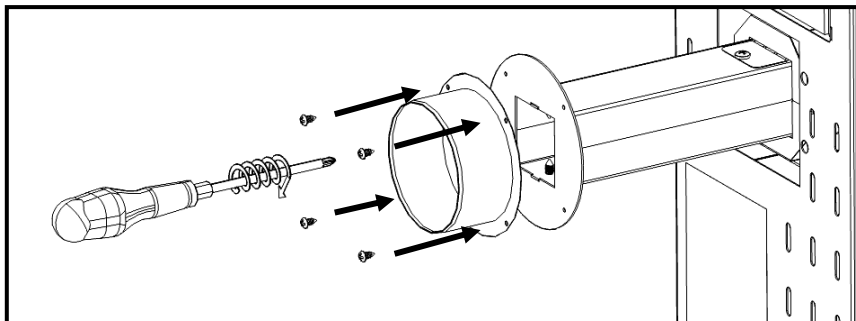
Figura 114 – Colocación de la boca de salida de aire en la estufa
