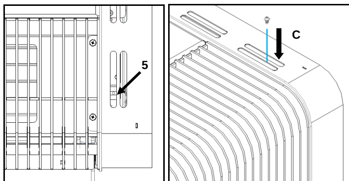
Figura 88 – Fijación de las envolventes Aspen
