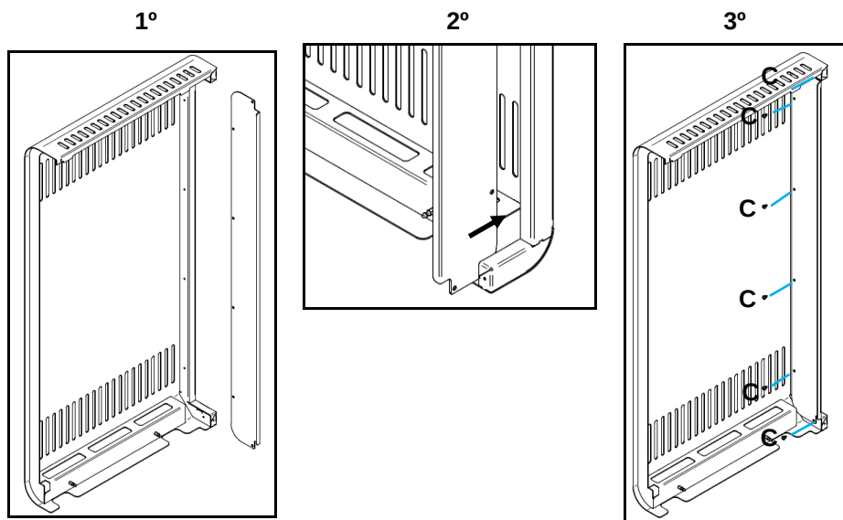
Figura 42 - Unión de la envolvente con la pieza frontal
