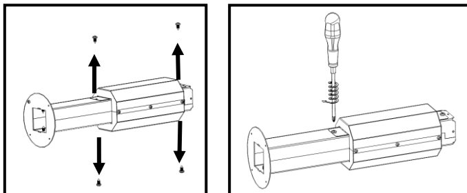
Figura 118 – Desmontaje del aislamiento térmico
