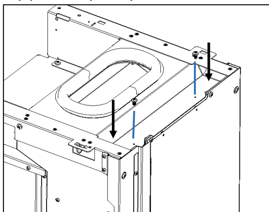
Figura 49 - Colocar los tornillos en lo depósito de pellets
