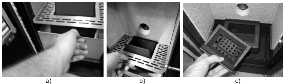
Figura 137 – a) Cestillo de quemado b) Rejilla; c) Cestillo de cenizas
