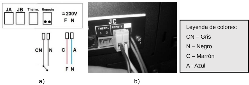
Figura 146 – Conexión del control remoto
