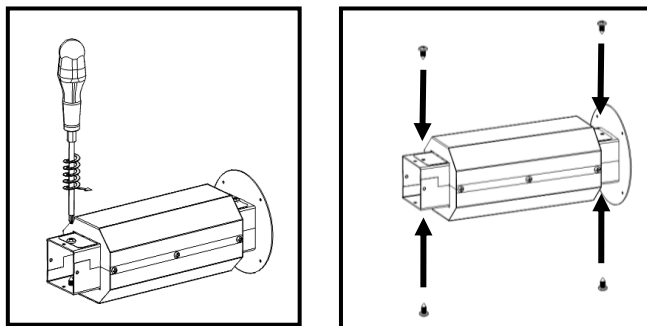
Figura 120 – Montaje del aislamiento térmico
