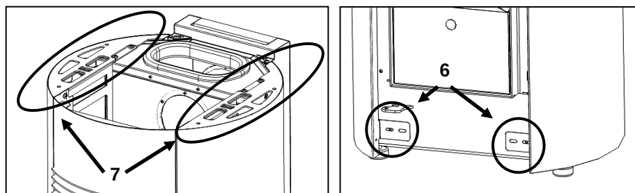
Figura 78 - Montaje de la tapa lateral
