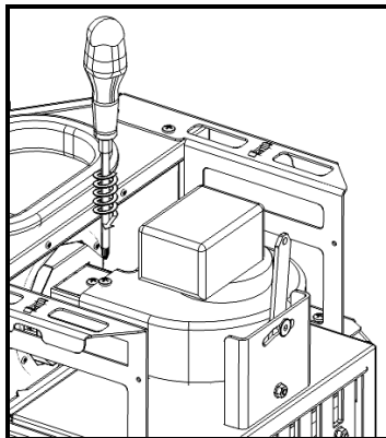
Figura 113 – Colocación de la guía de aire en la estufa
