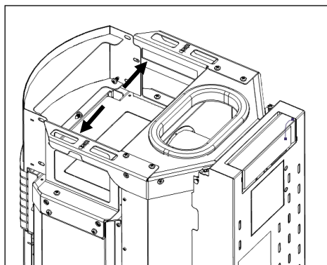
Figura 74 - Fijación frontal
