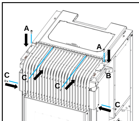
Figura 101 – Apriete de la rejilla frontal
