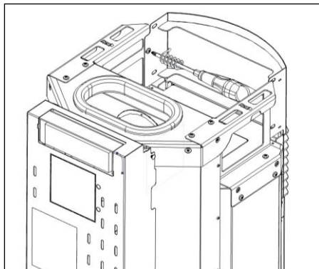
Figura 74 - Fijación frontal
