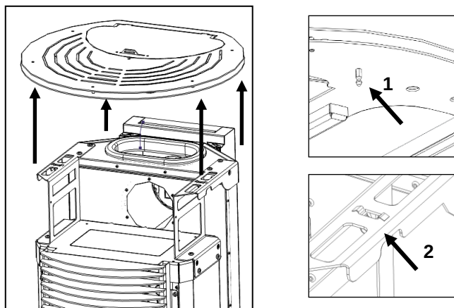
Figura 72 - Desmontaje de la parte superior del K500
