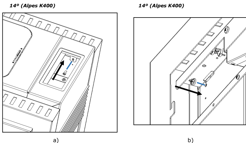
Figura 65 A y B – Fijación dos lados
