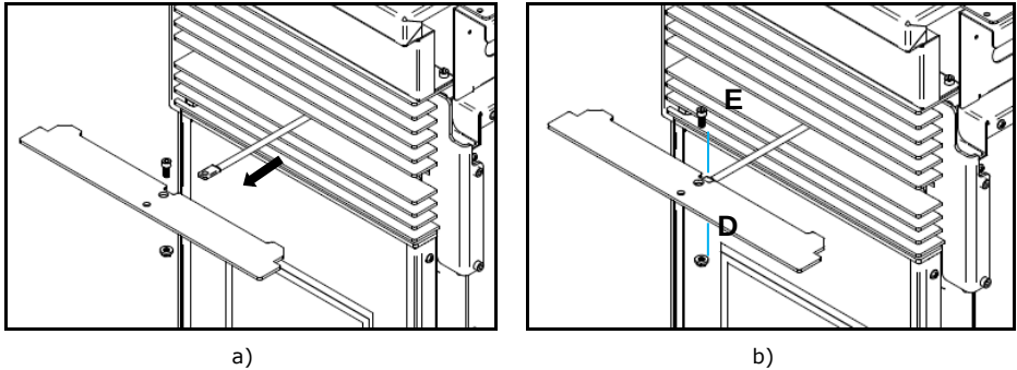
Figura 38 - Pala de agarre de registro
