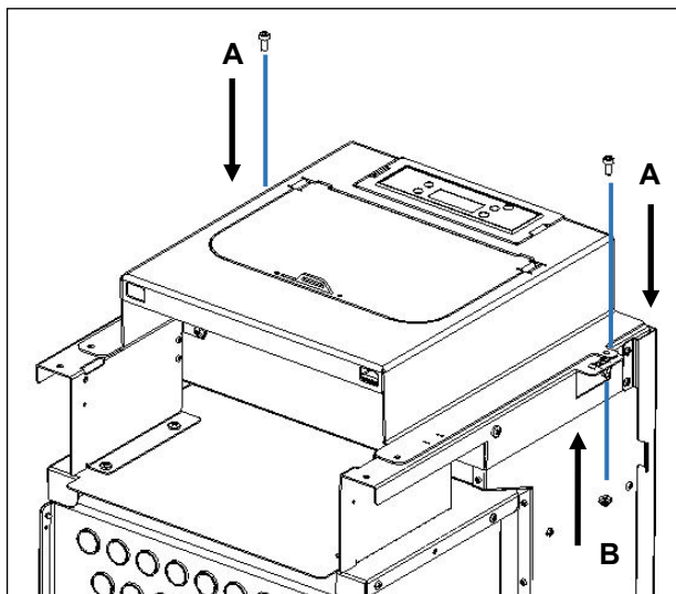
Figure 54 - La fixation à la partie supérieure de la structure de l'équipement
