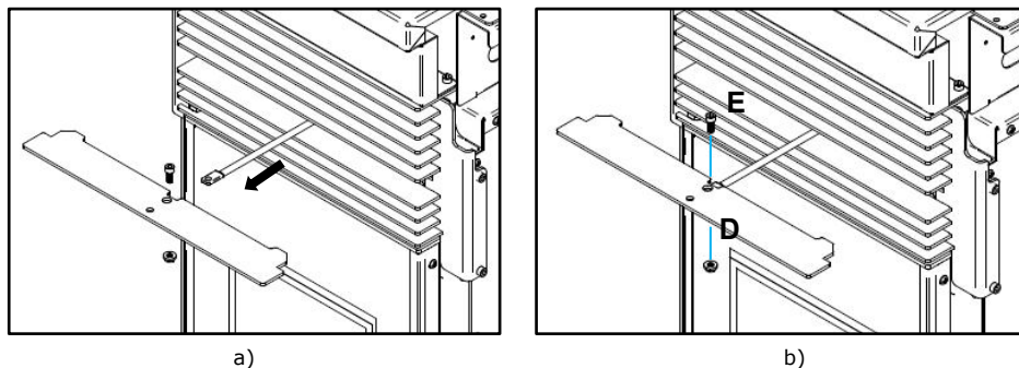
Figure 38 - Fixation de la plaque mobile à la tige de nettoyage
