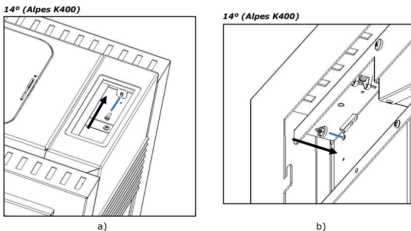
Figure 65 A e B - Fixation des côtés structurels
