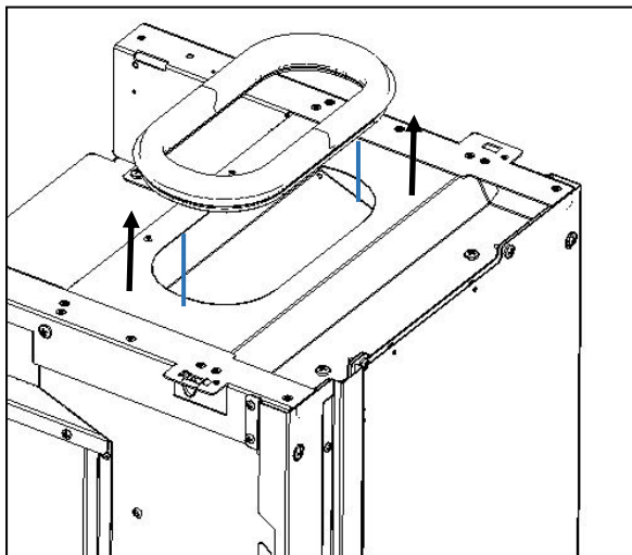
Figure 50 - Enlèvement du joint en caoutchouc dans la machine
