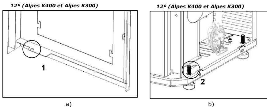
Figure 62 - Emboitement inférieur des structures latérales
