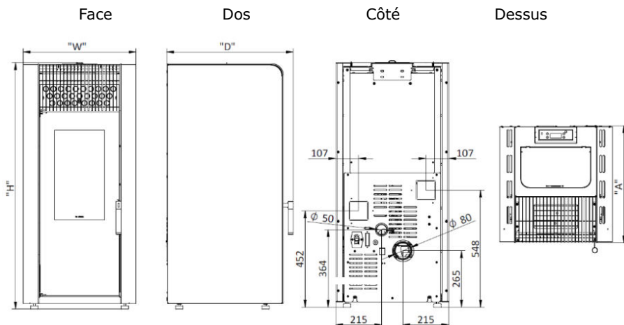
Figure 2-D – Dimensions du poêle à granulés K600 (exemple modèle Aspen)
