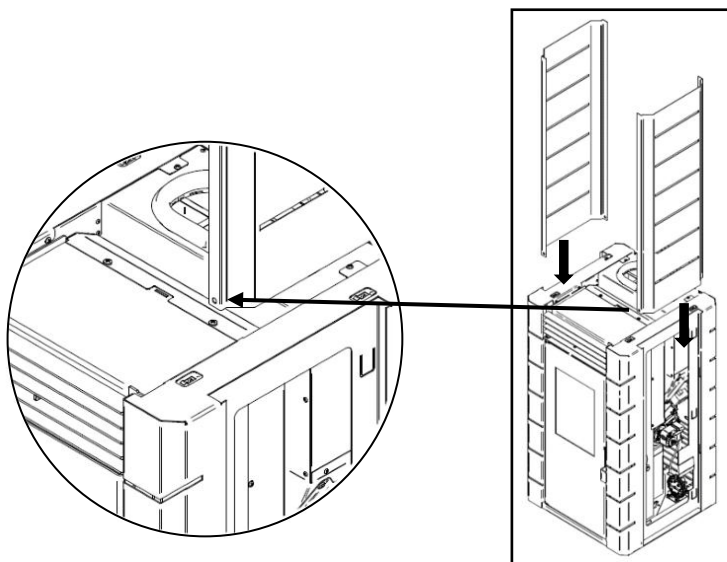
Figure 25 - Mise en place des panneaux latéraux
