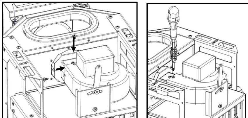
Figure 113 - Fixation du guide d'air sur le poêle
