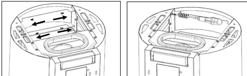
Figure 79 - Fixation du couvercle à l'avant de la finition
