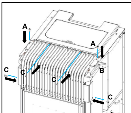
Figure 86 - Installation de la grille avant
