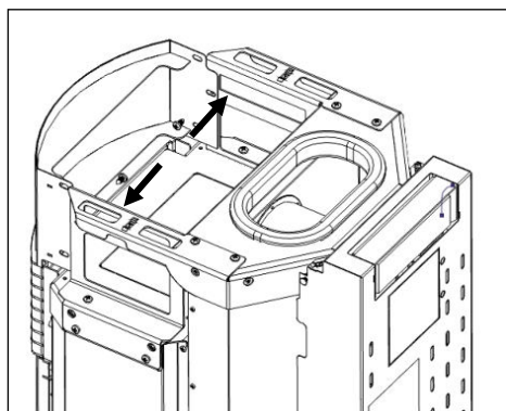
Figure 74 - Fixation de la façade de finition
