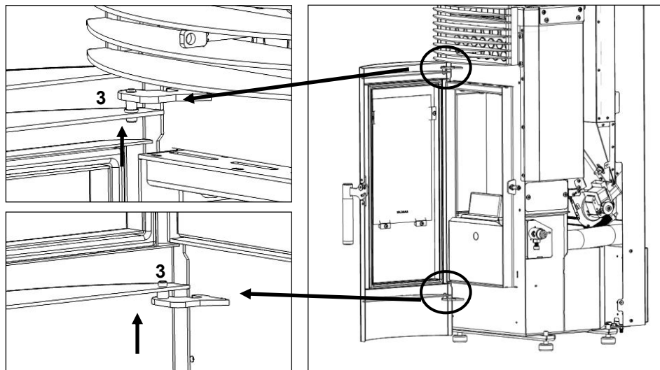
Figure 75 - Retrait de la porte
