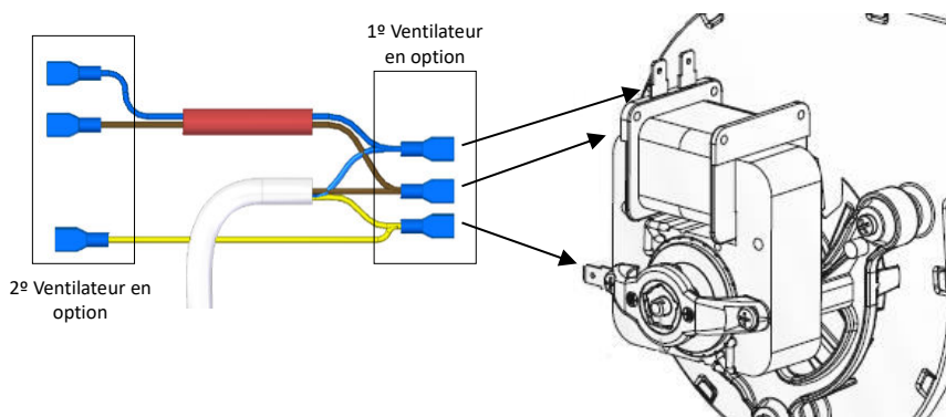
Figure 132 - Raccordement électrique au ventilateur
