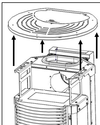
Figure 72 - Démontage de la partie supérieure du K500
