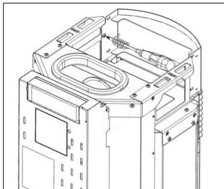
Figure 74 - Fixation de la façade de finition
