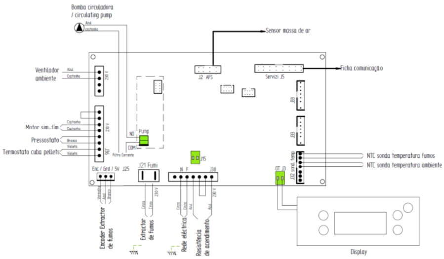
Figura 69 - Esquema eléctrico Hidro 1 e 23
