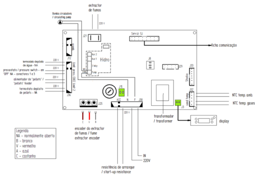
Figura 68 - Esquema eléctrico Hidro 12
