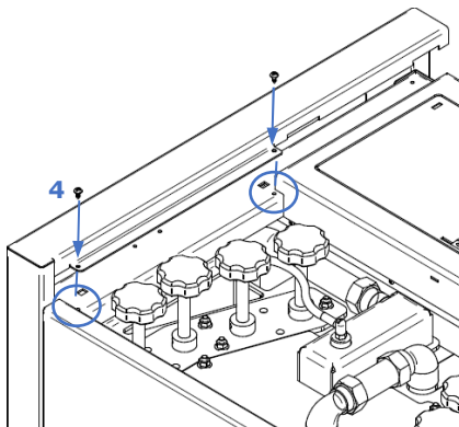
Figura 36 – Colocação das envoltentes Hidro 17 e Hidro 23
