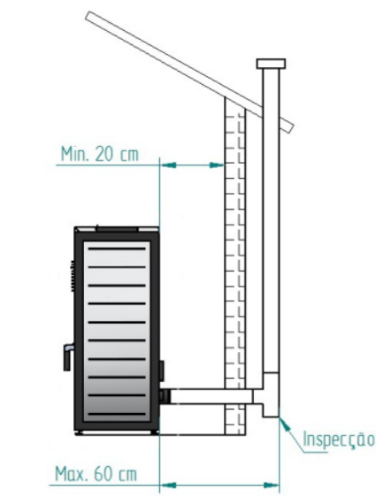
Figura 10 – Vista lateral da instalação sem chaminé, com exemplo do ponto de inspecção
