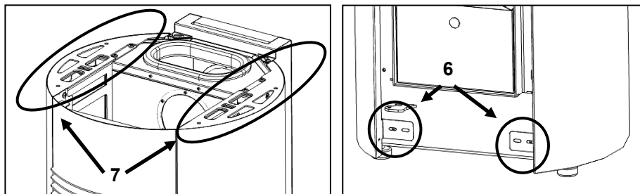
Figure 48 – Montage du couvercle latéral
