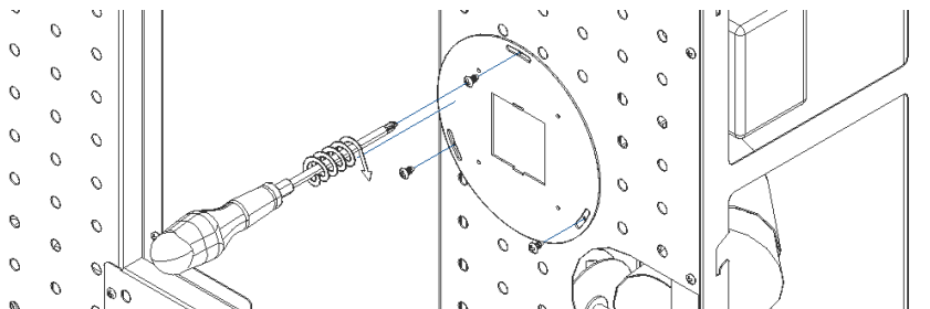
Figure 62 – Fixation du guide
