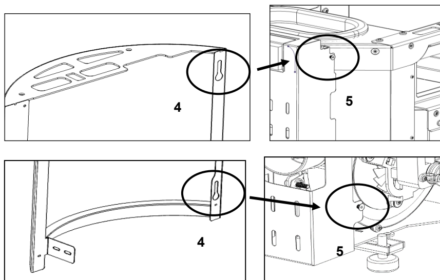
Figure 47 – Montage du couvercle latéral
