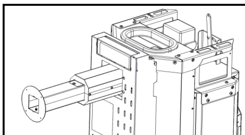
Figure 77 – Guide d'air
