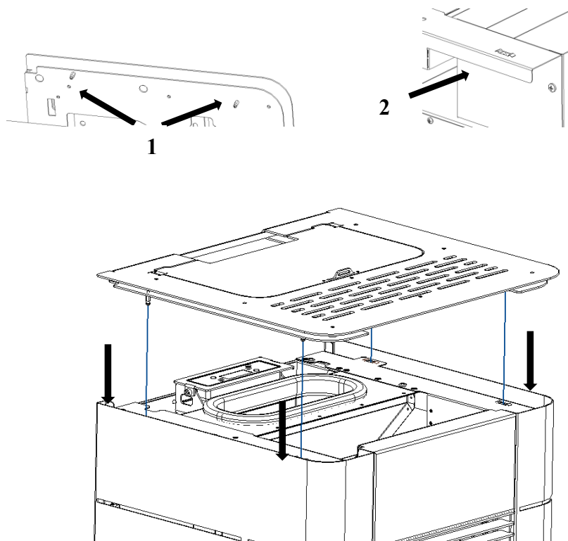
Figure 39 – Emboîtement du panneau supérieur
