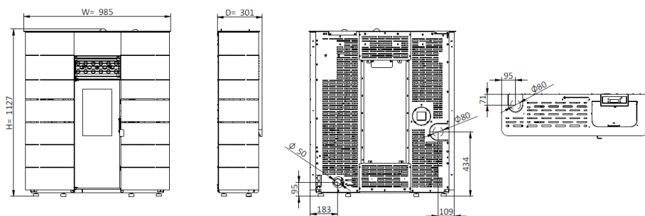
Figure 2-A – Dimensions du poêle granulés Nevada
