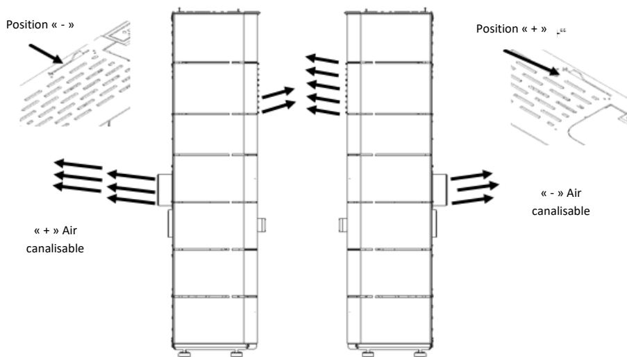
Figure 86 – Réglage du registre d'air canalisable "+" ou "-"
