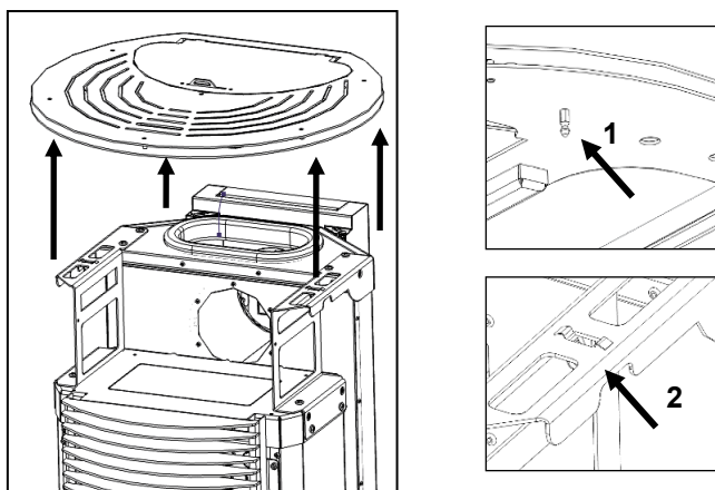
Figure 42 – Enlèvement de la partie supérieure de l'appareil K500
