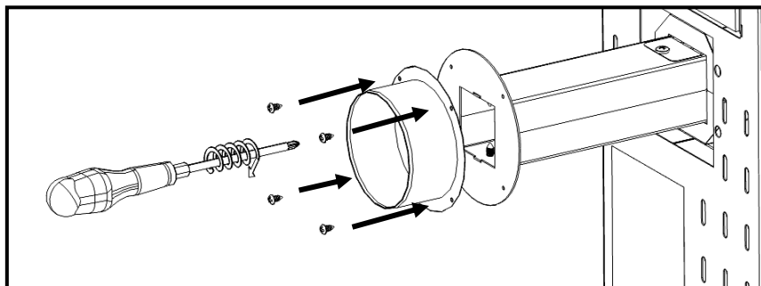
Figure 79 – Fixation buse sortie d'air
