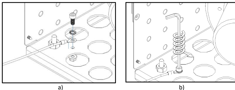
Figure 64 – Connexion câble de terre du ventilateur
