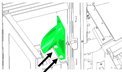
Figure 110 – Retrait du canal d'alimentation
