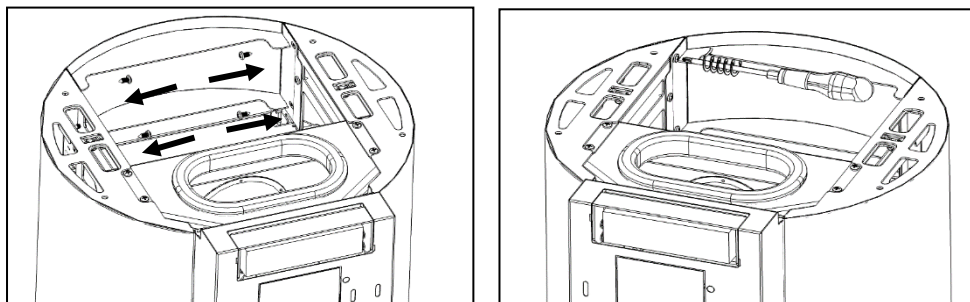
Figure 49 – Fixation du couvercle à l'avant de la finition
