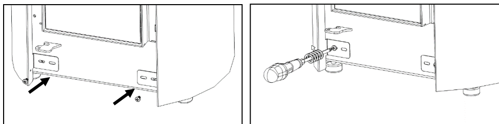
Figure 50 – Fixation du couvercle à l'avant de l'appareil
