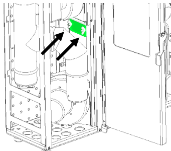
Figure 108 – Couvercles à enlever dans l'équipement
