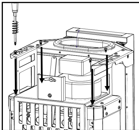
Figure 75 – Fixation ventilateur
