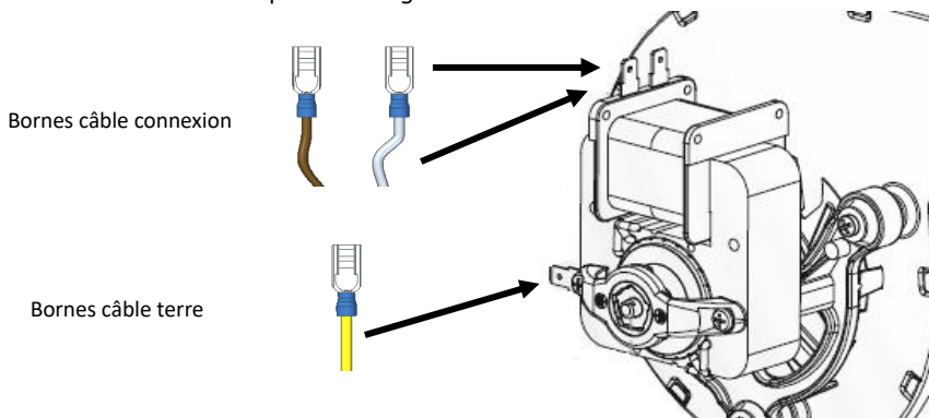
Figure 81 – Raccordement électrique au ventilateur
