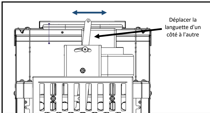
Figure 82 – Vérifier le verrouillage du registre
