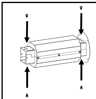
Figure 85 – Remontage de l'isolation thermique
