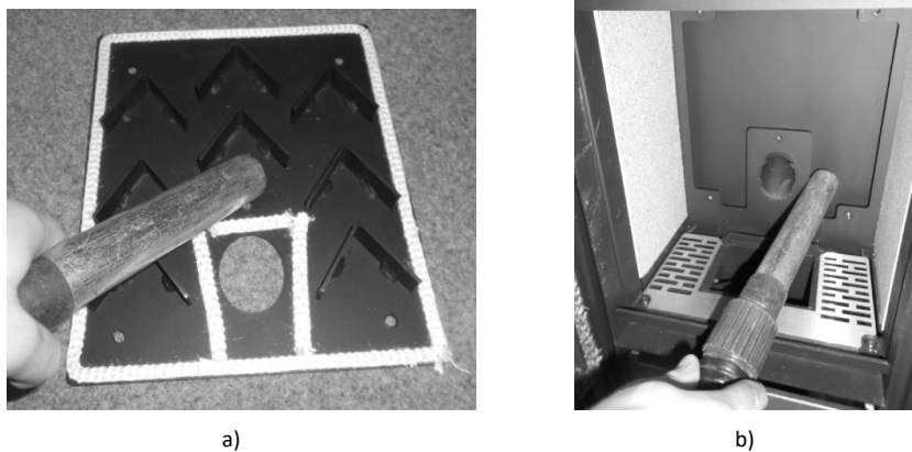
Figure 114 – Nettoyage du circuit de fumée
