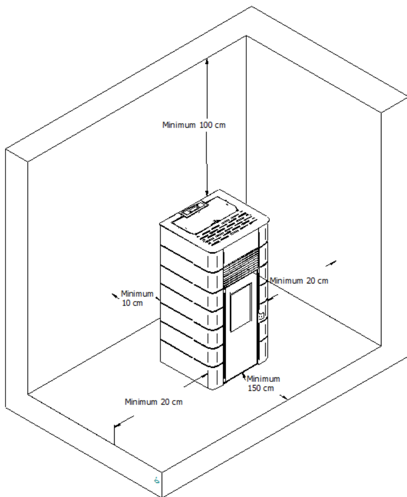
Figure 7 – Distance minimale de toutes les surfaces Everest
