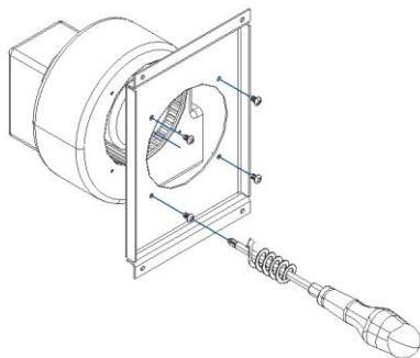
Figure 58 – Support de fixation avec ventilateur
