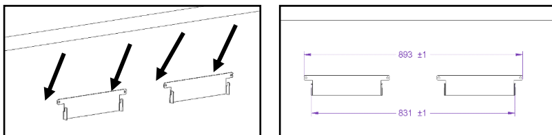
Figure 91 – Support de fixation C et dimensions à respecter
