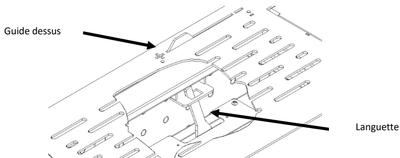
Figure 68 – Emboîtement du dessus sur le registre d'entrée d'air canalisable
