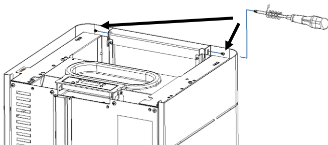
Figure 38 – Emboîtement des panneaux latéraux
