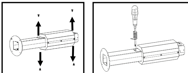
Figure 83 – Démontage de l'isolation thermique
