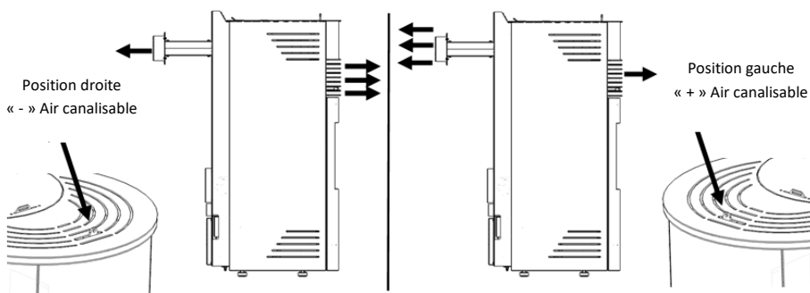
Figure 87 – Réglage du registre d'air canalisable "+" ou "-"
