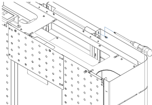
Figure 32 – Fixation des couvercles latéraux
