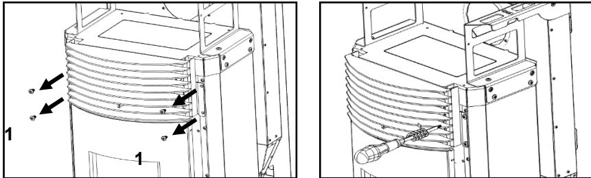
Figure 71 – Retrait grille latérale
