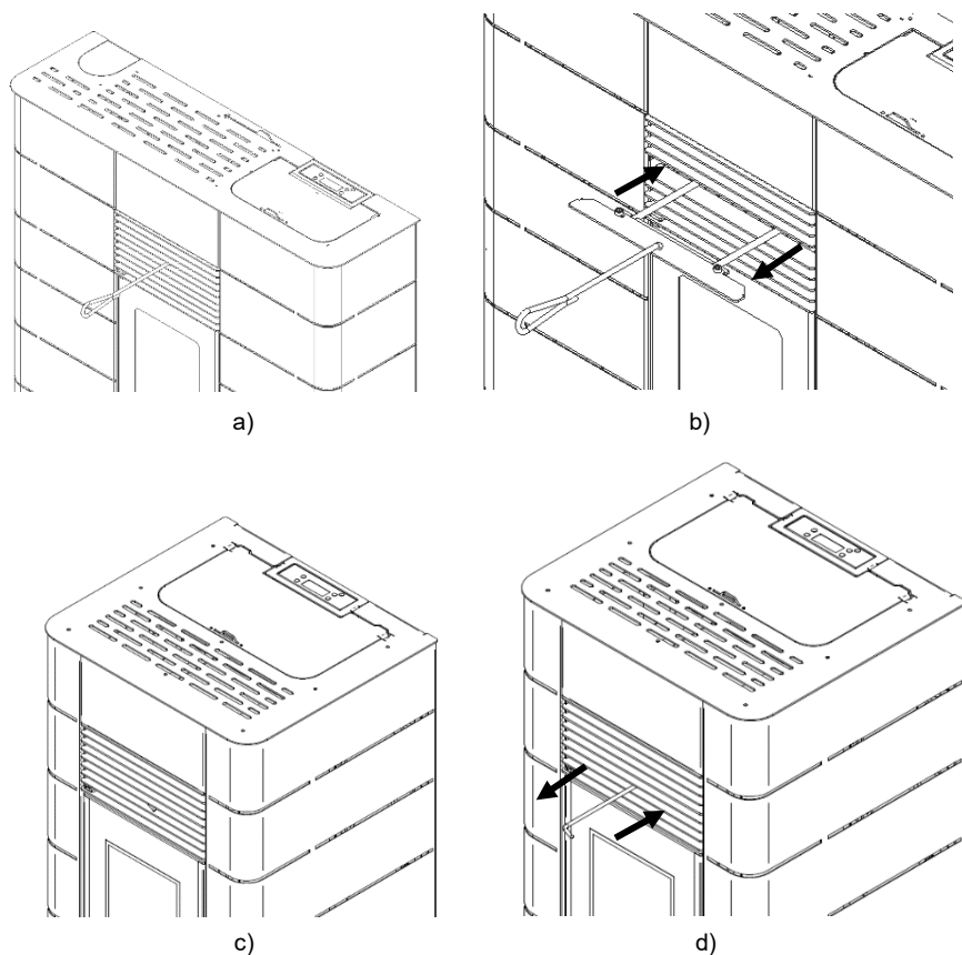
Figure 104 – Barre de nettoyage de l'échangeur
