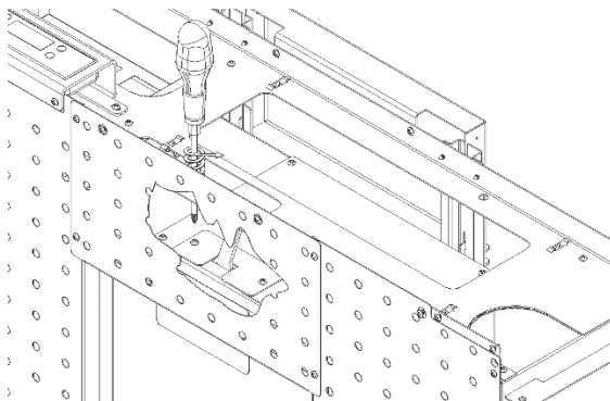
Figure 67 – Enlèvement couvercle de blocage
