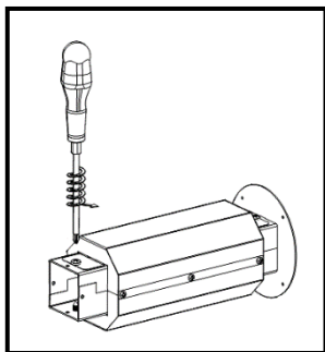
Figure 85 – Remontage de l'isolation thermique
