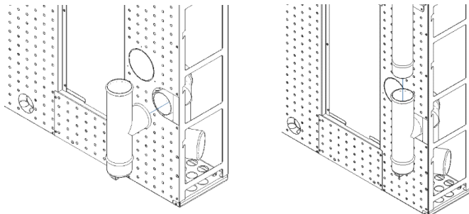
Figure 17 – Raccord du T et tuyau d'échappement option 2
