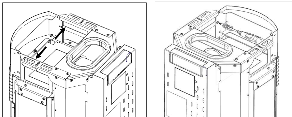
Figure 44 – Fixation de la façade de finition
