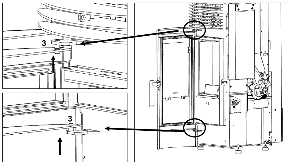
Figure 45 – Démontage de la porte
