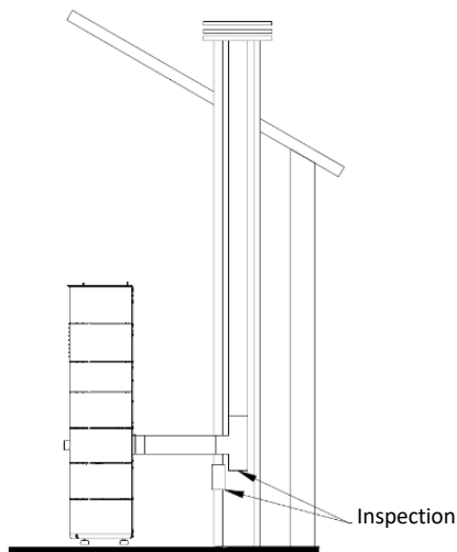
Figure 26 – Vue latérale de l'installation avec cheminée, avec exemple du point de contrôle
