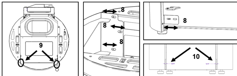
Figure 51 – Réglage des habillages
