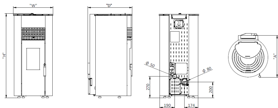
Figure 2-C – Dimensions du poêle granulés K500 (exemple Amazon)
