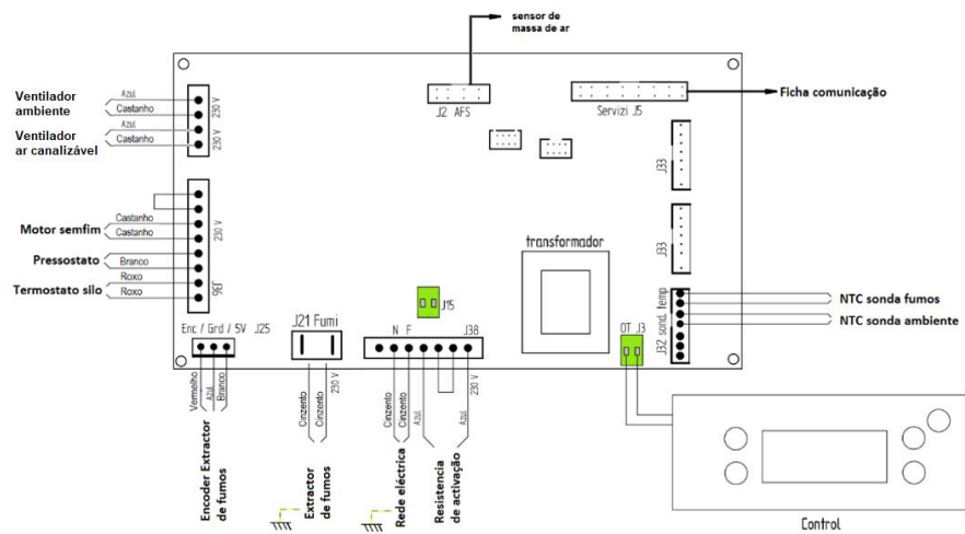
Figure 127 – Schéma électrique
