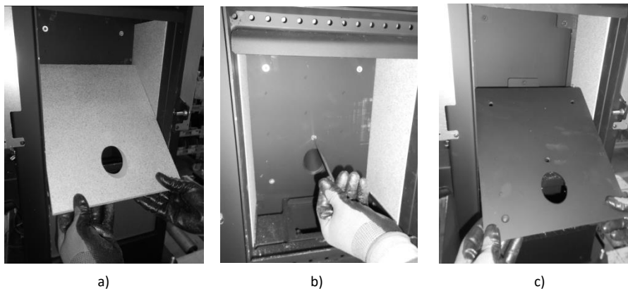
Figure 113 – Retrait du circuit de fumée
