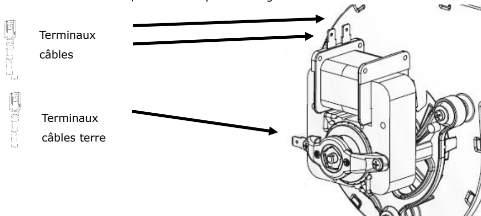
Figure 66 – Connexion câblage au ventilateur
