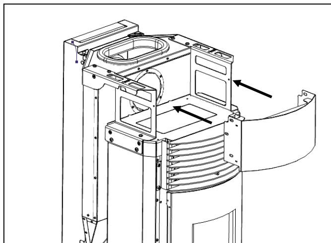
Figure 43 – Fixation avant du cadre
