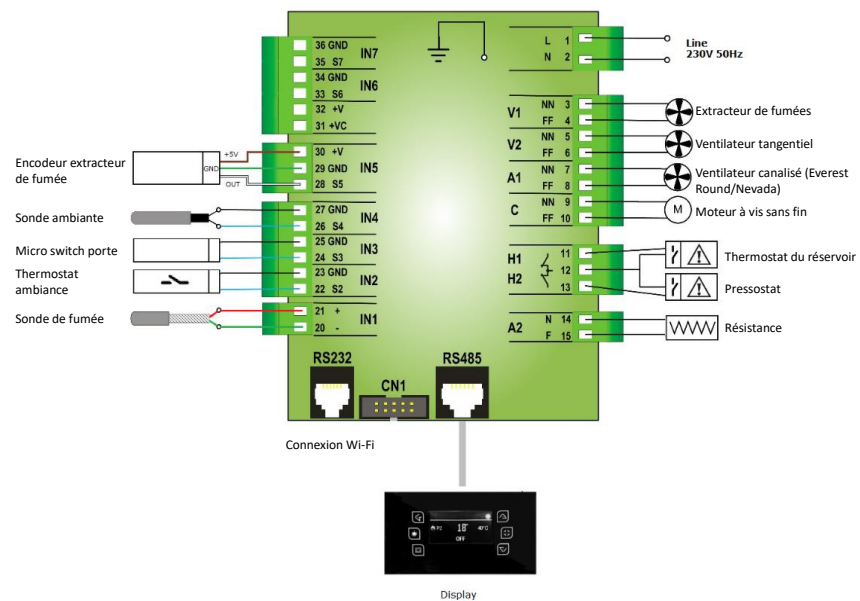
Figure 128 – Schéma électrique Columbus
