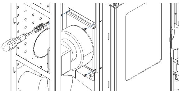
Figure 59 – Fixation du ventilateur sur l'équipement
