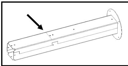
Figure 84 – Zone de coupe de la partie "guide" de l'air de la tuyauterie
