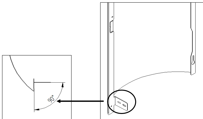
Figure 46 – Angle de l'onglet inférieur
