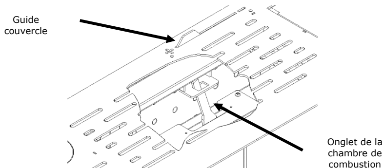
Figure 33 – Clapet d'air canalisable
