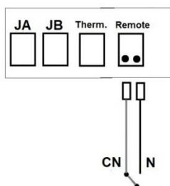
Figura 120 - Ligações do comando externo com fios
