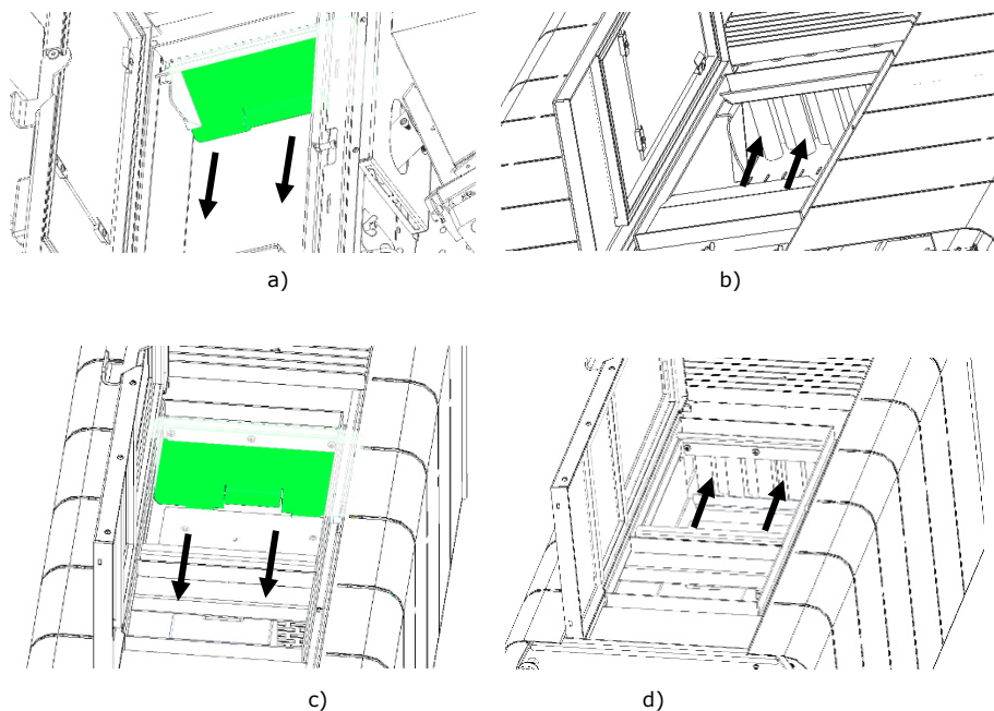
Figura 112 - Remoção chapa defletora e limpeza permutador
