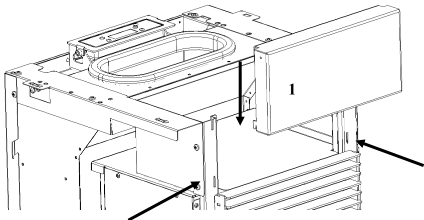
Figura 35 - Encaixe frontal das envolventes
