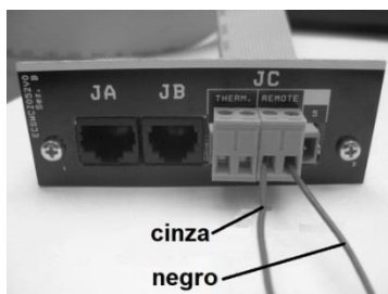
Figura 120 - Ligações do comando externo com fios
