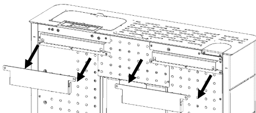
Figura 92 - Colocação do equipamento nos apoios fixos na parede
