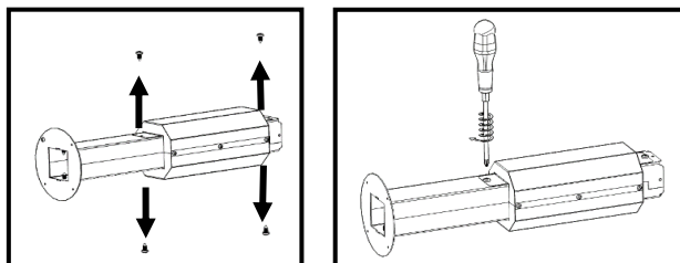
Figura 83 - Desmontagem do isolamento térmico
