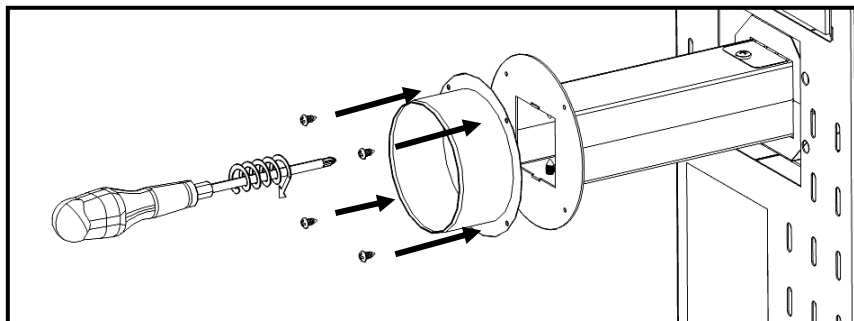
Figura 79 - Fixação boca saída de ar na salamandra
