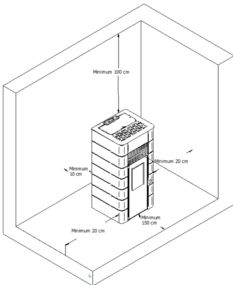
Figura 7 - Distâncias mínimas de todas as superfícies Everest
