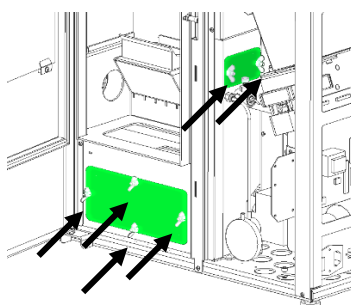
Figura 108 - Tampas a retirar no equipamento
