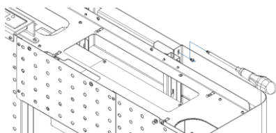
Figura 55 - Remoção parafuso capa lateral
