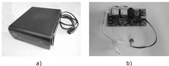
Figura 122 - a) Exemplo de UPS (não incluído no kit); b) componentes do kit UPS
