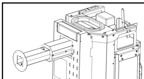
Figura 77 - Encaixe guia ar na salamandra
