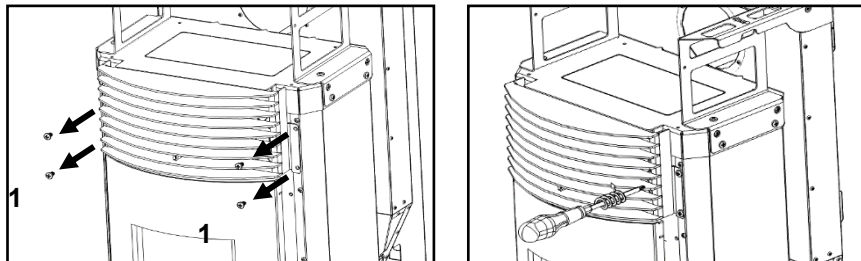
Figura 71 - Remoção da grelha lateral
