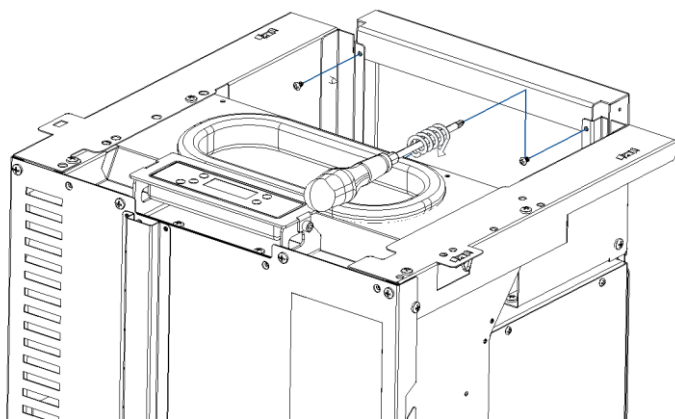
Figura 36 - Fixação frontal das envolventes
