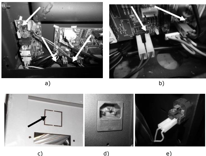
Figura 123 - Instalação do kit UPS
