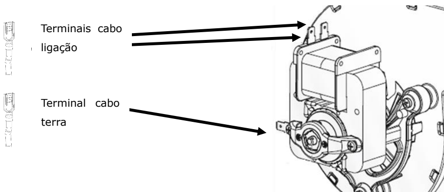
Figura 66 - Ligação cablagem ao ventilador
