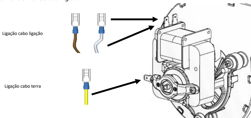
Figura 81 - Ligação cablagem ao ventilador
