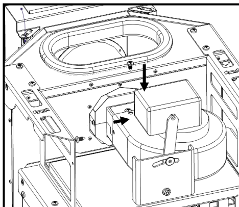
Figura 78 - Fixação guia ar na salamandra
