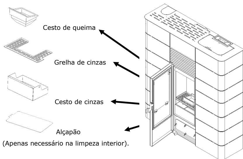
Figura 105 - Acessórios a retirar na limpeza do equipamento
