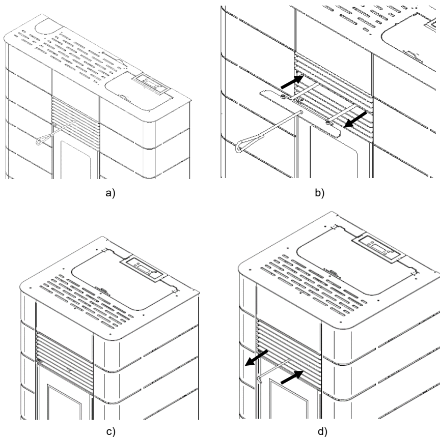
Figura 104 - Barra de limpeza do permutador
