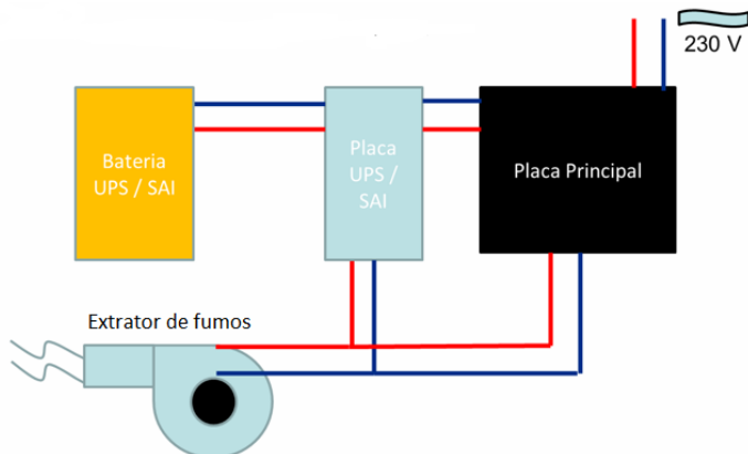
Figura 124 - Esquema funcionamento Kit UPS
