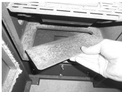
Figura 107 - Limpeza do interior da salamandra
