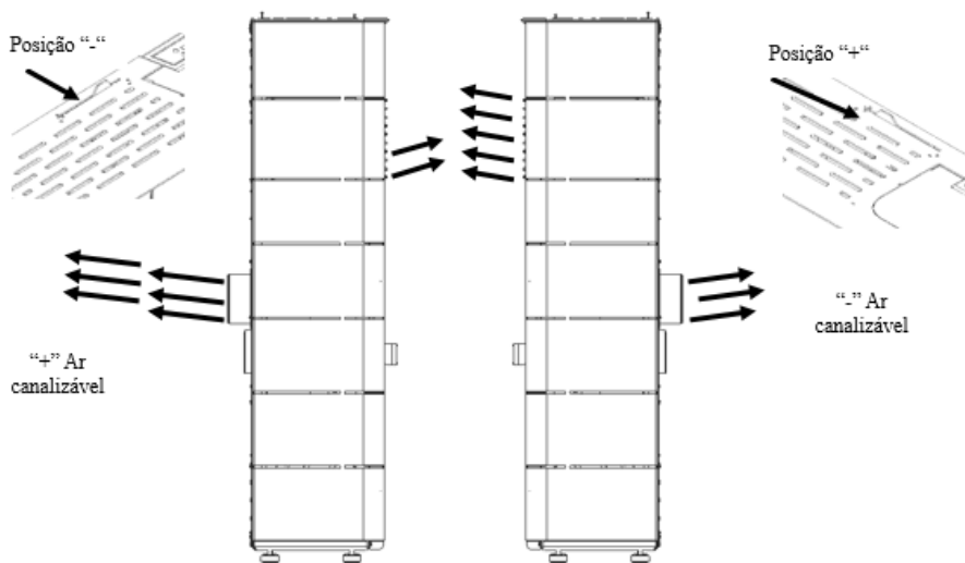
Figura 86 - Regulação do registo do Ar canalizável "+" ou "-"
