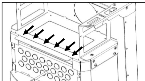
Figura 73 - Remoção pala frontal
