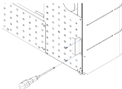
Figura 90 - Fixação dos apoios D
