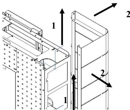
Figura 56 - Remoção capa lateral
