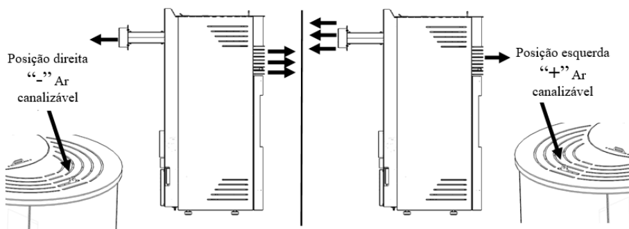
Figura 87 - Regulação do registo do Ar canalizável "+" ou "-"
