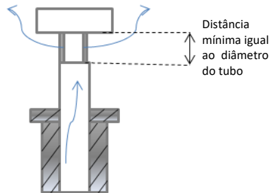
Figura 29 - União correta
