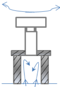
Figura 28 - União incorreta
